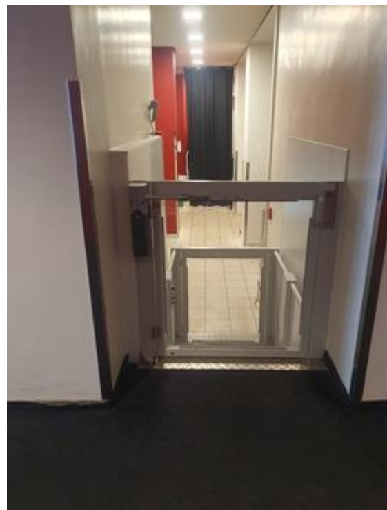
Abbildung 4: Derselbe Hublift von der oberen Ebene aus. Sichtbar sind der Fliesenboden des Foyers (untere Ebene) und der feste Teppichboden (obere Ebene)
